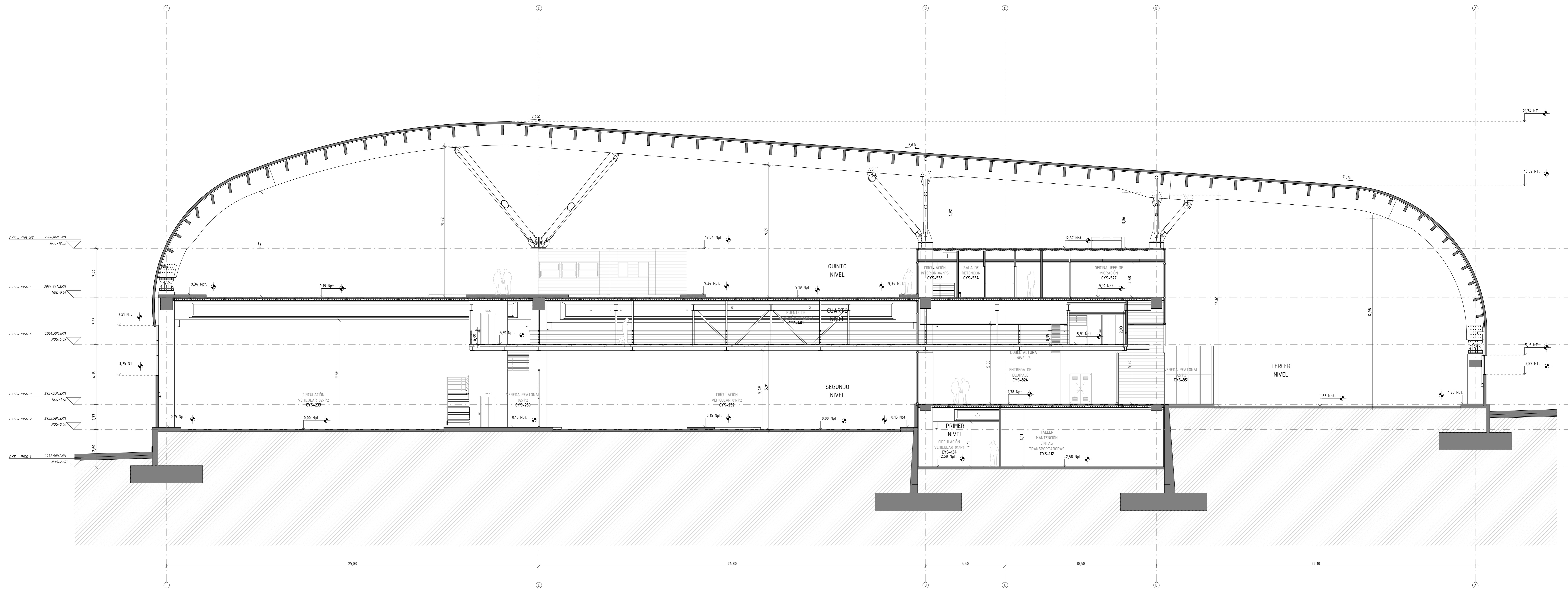
2 | CORTE TRANSVERSAL 2 1 : 100
